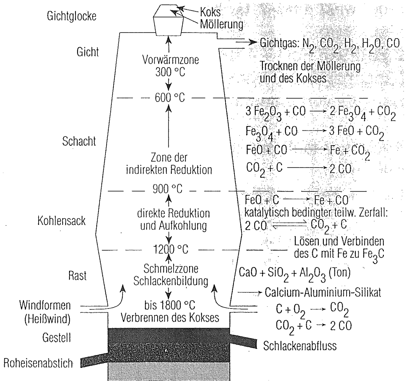
Abb. 4.3.4-2 Hochofen
