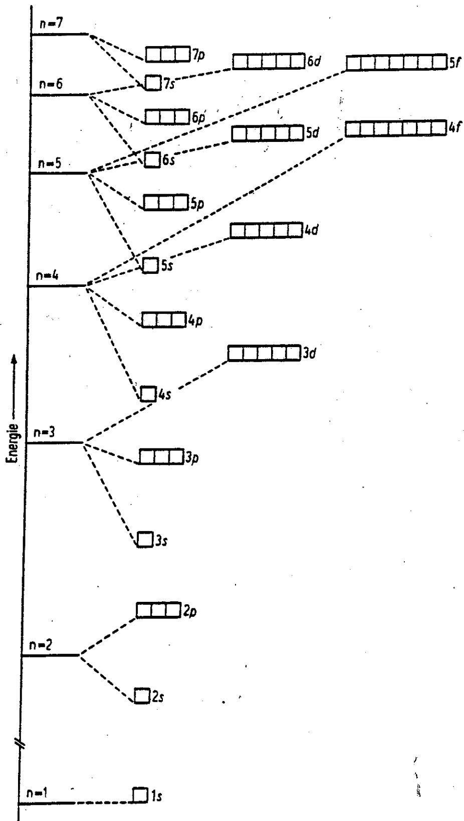
Abb. 1.5. Energieniveaudiagramm von Atomorbitalen.
