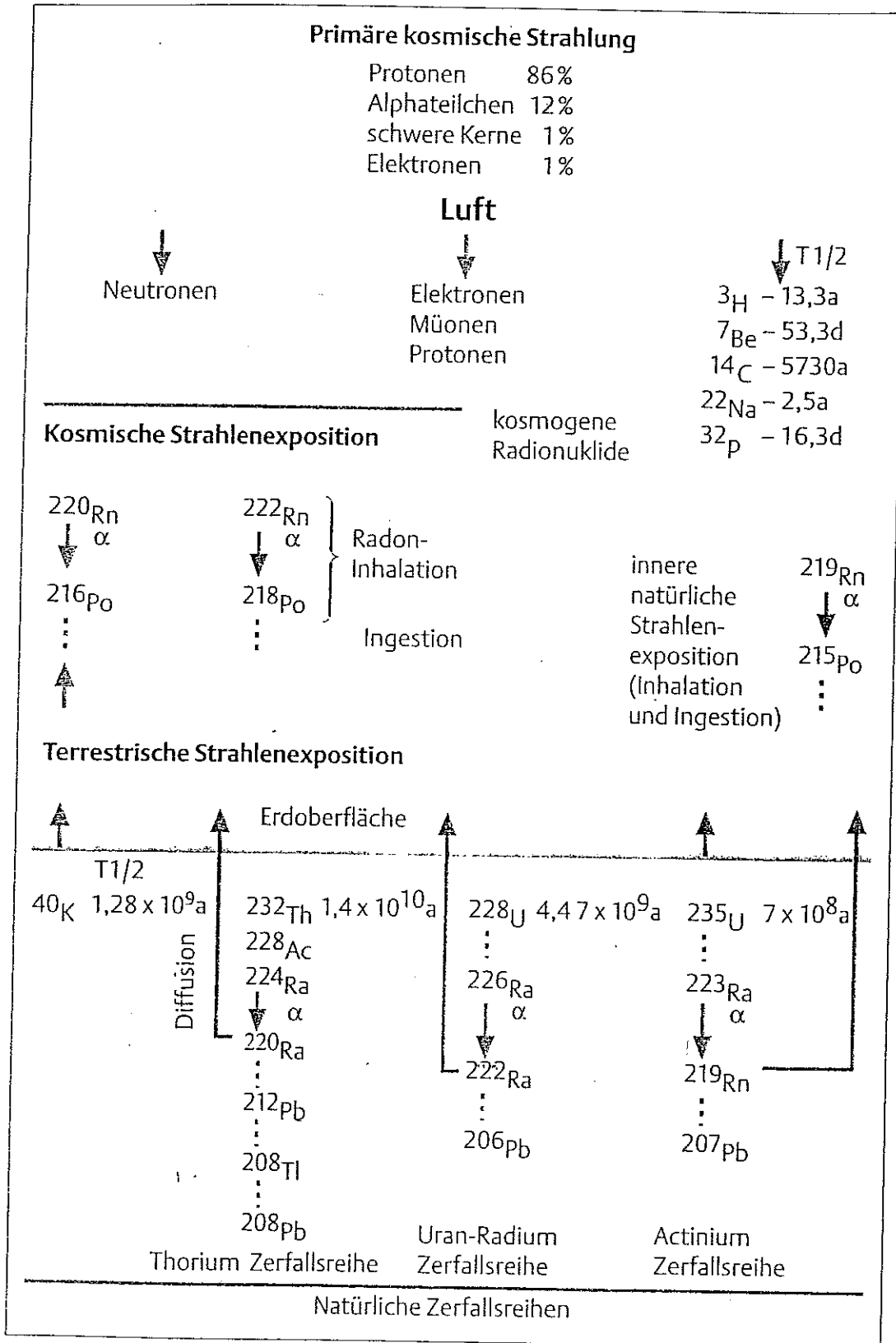
Abb. 9.6 Natürliche Strahlenexposition; a = Jahr, d = Tag
